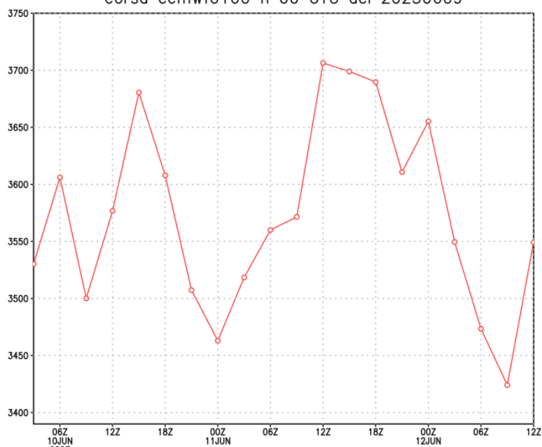
Zero termico Ancona corsa ecmwf0100 h 00 UTC del 20230609
