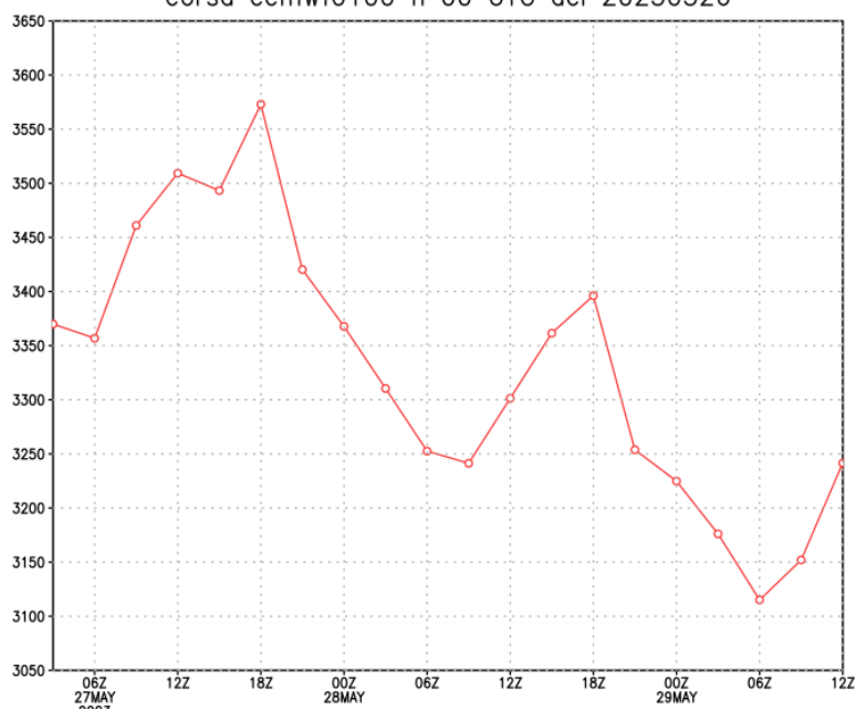
Zero termico Ancona corsa ecmwf0100 h 00 UTC del 20230526
