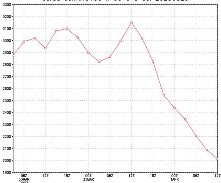
Zero termico Ancona corsa ecmwf0100 h 00 UTC del 20230329
