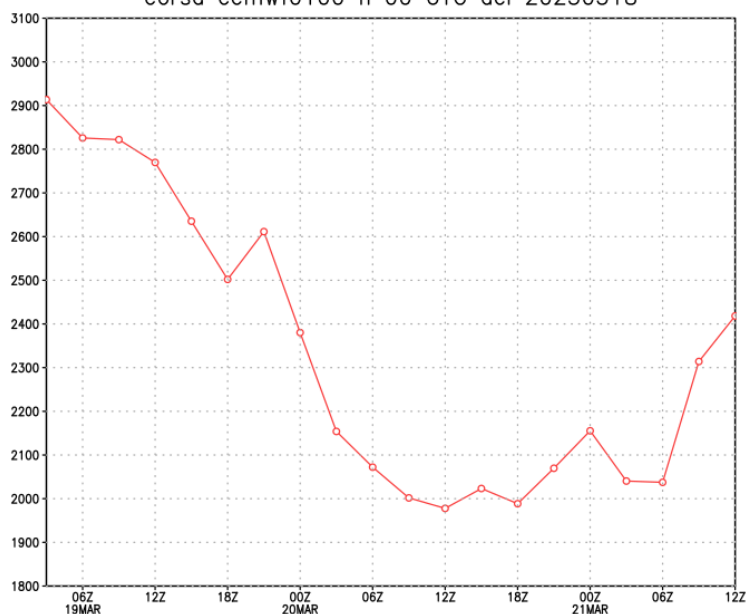
Zero termico Ancona corsa ecmwf0100 h 00 UTC del 20230318
