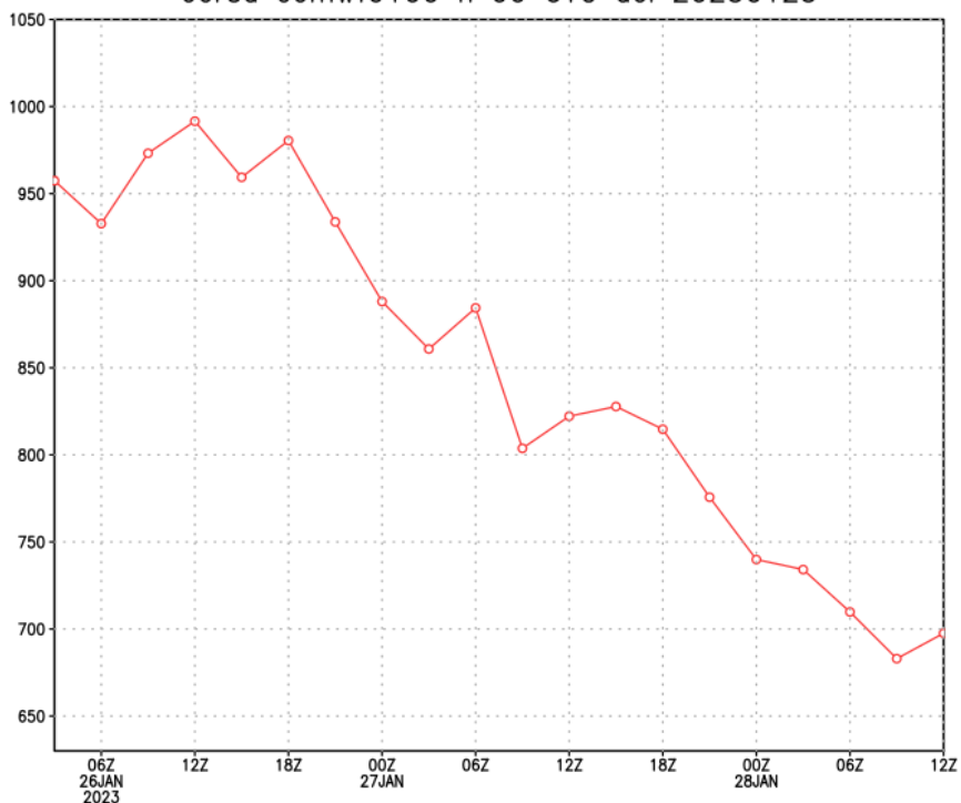
Zero termico Ancona corsa ecmwf0100 h 00 UTC del 20230125
