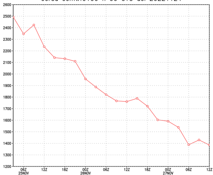
Zero termico Ancona corsa ecmwf0100 h 00 UTC del 20221124
