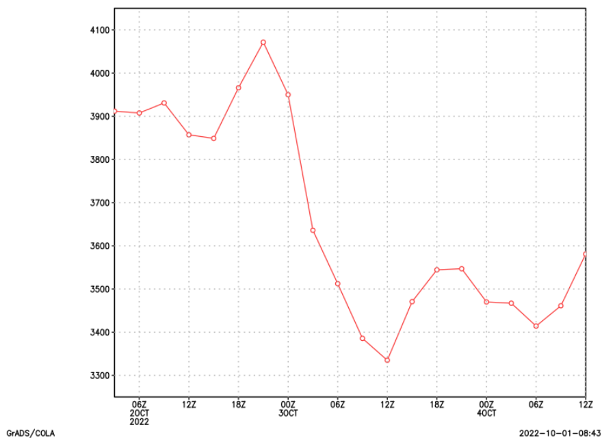
Zero termico Ancona corsa ecmwf0100 h 00 UTC del 20221001
